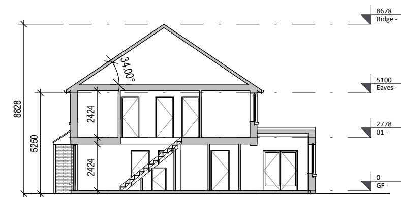
7 Section B-B 1 : 200
