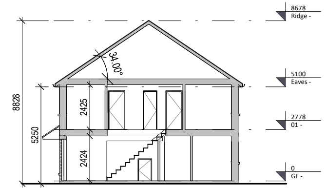
6 Section A-A 1 : 200
